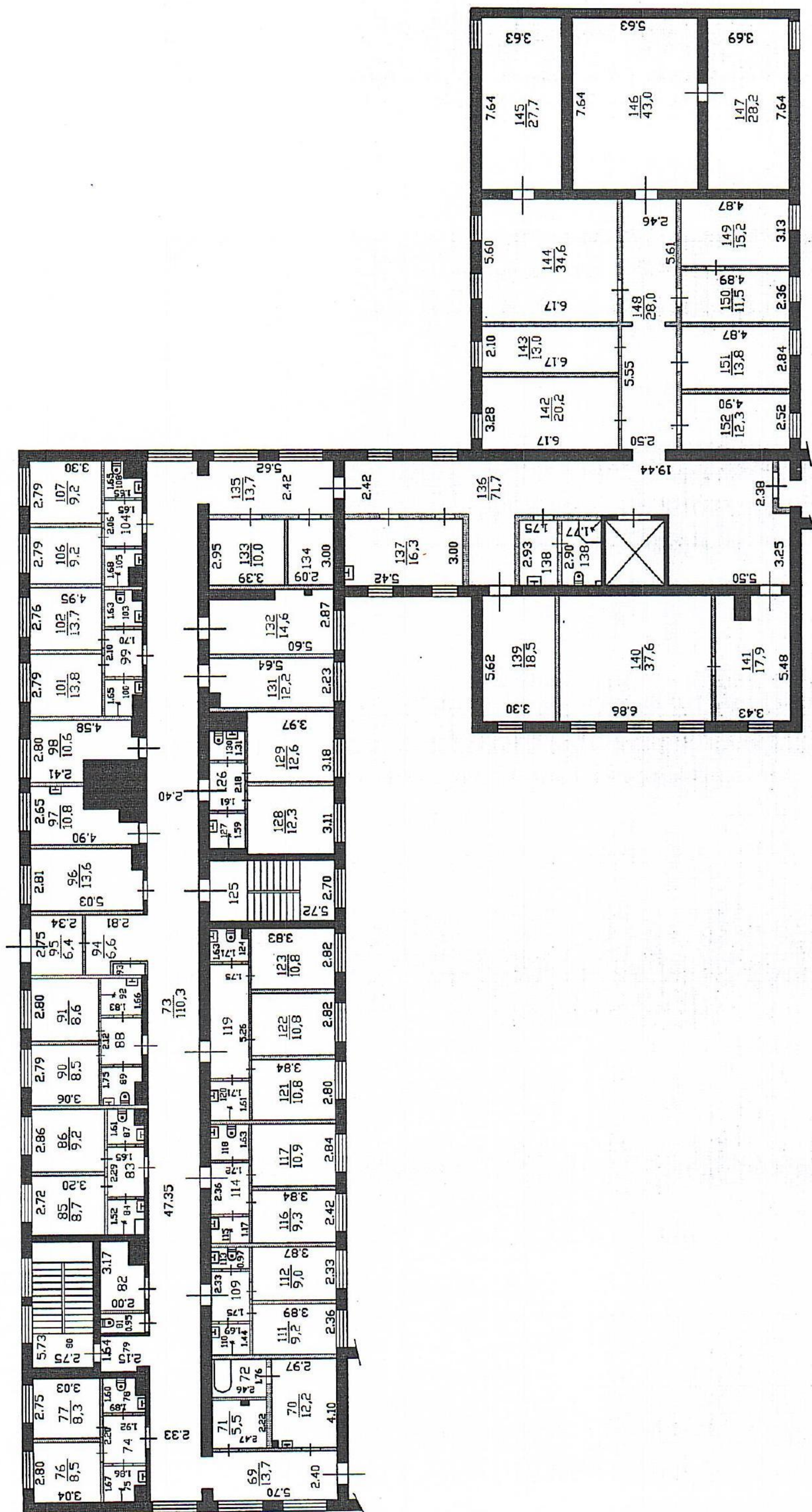
ПЛАН 2-ГО ЭТАЖА
